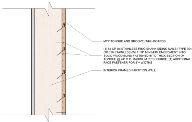
1.0 MTP TONGUE & GROOVE
