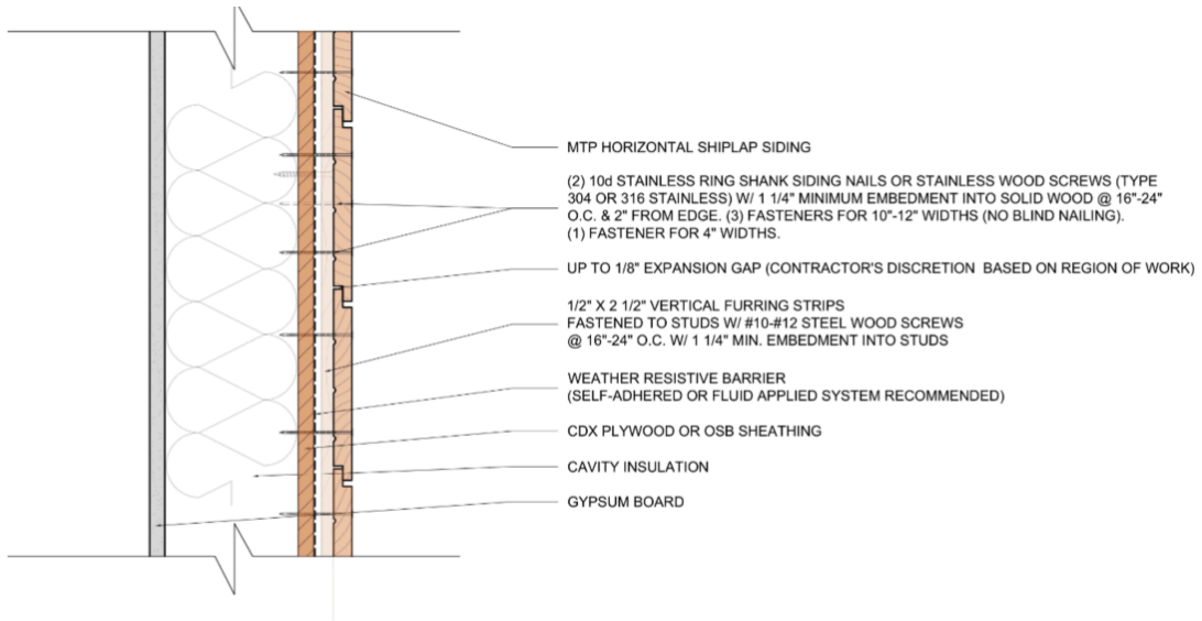
○ MTP HORIZONTAL SHIPLAP
